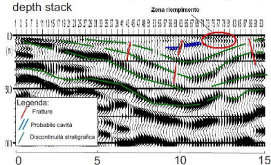
ALL 2:Sismica a riflessione: Sezione interpretata depth stack
